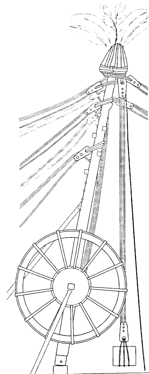
Kran vom Hateriergrab; Vatikan. Museen, Museum Gregoriano Profano (Inv. 9998), 120 n. Chr. (Zeichnung nach Relief mit Ergänzungen).
